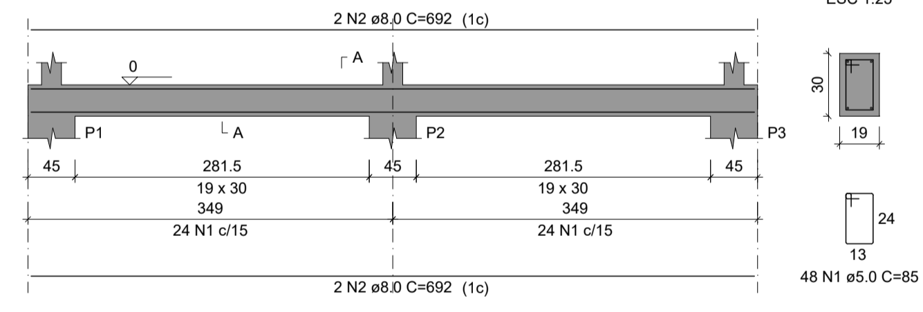
Vb3 ESC 1:50
