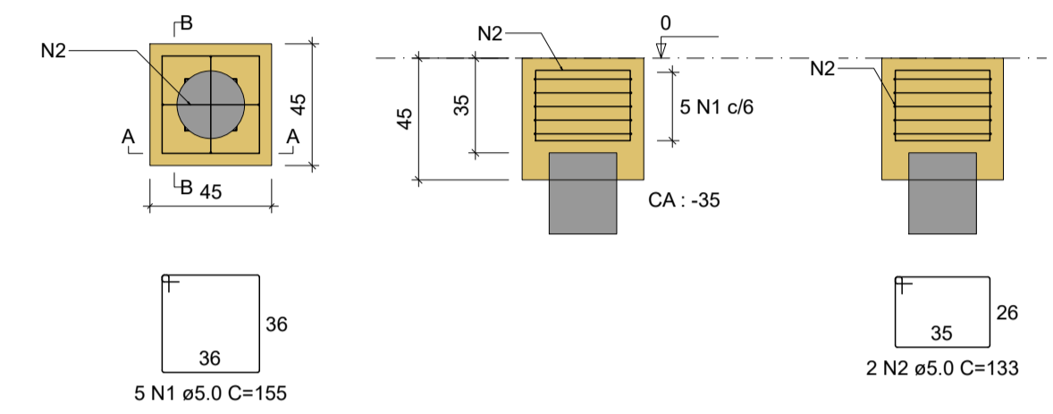
B6 1xD25-C30 PLANTA ESC 1:25
