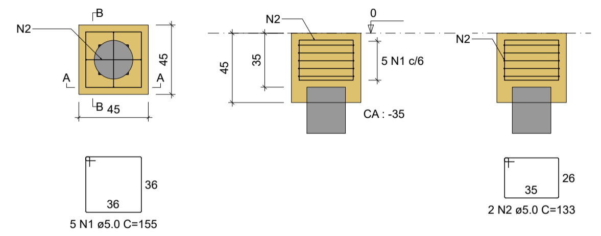
B8 1xD25-C30 PLANTA ESC 1:25
