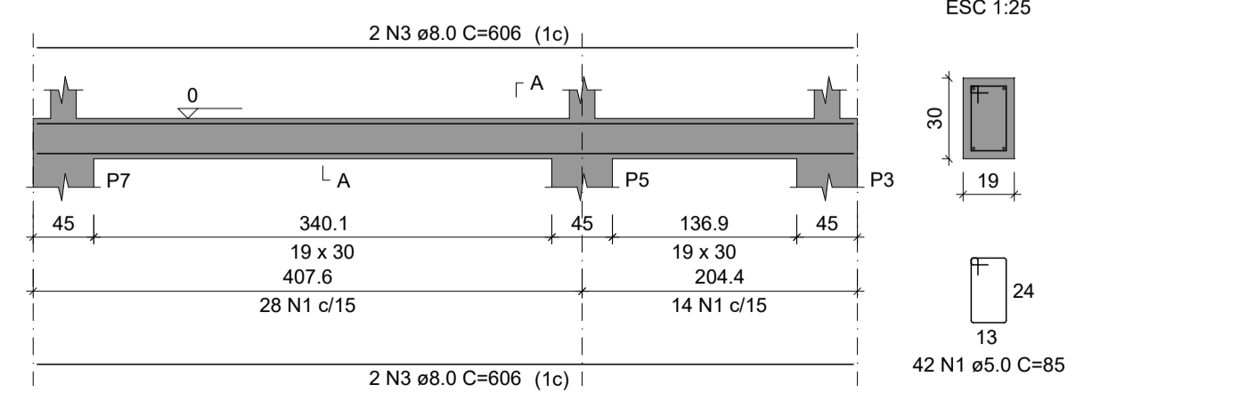
Vb6 ESC 1:50
