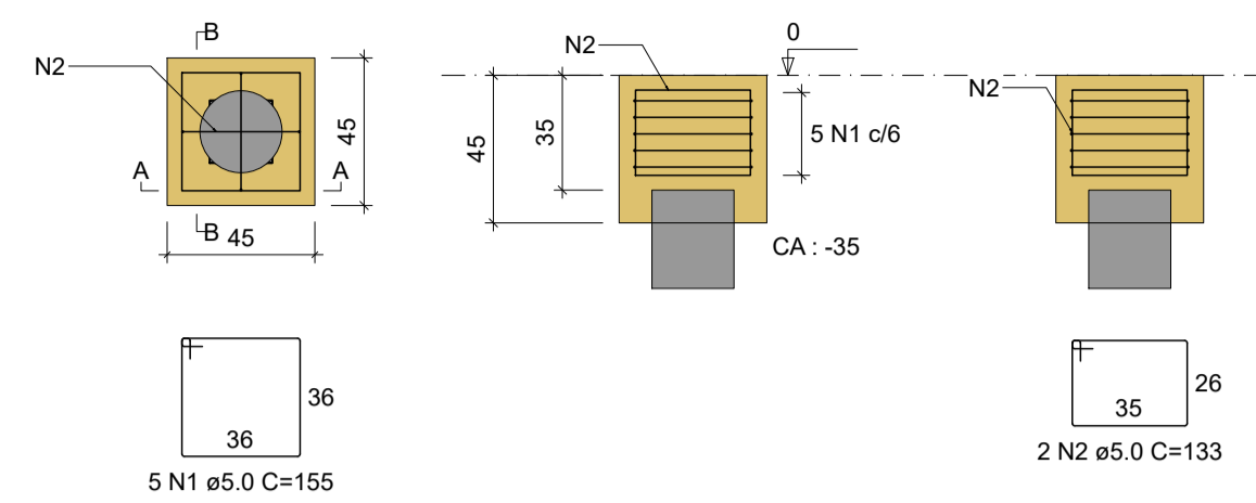
B5 1xD25-C30 PLANTA ESC 1:25
