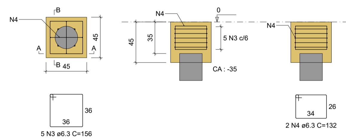
B9 1xD25-C30 PLANTA ESC 1:25
