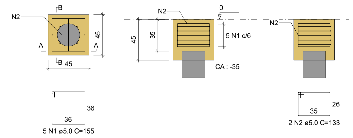
B7 1xD25-C30 PLANTA ESC 1:25
