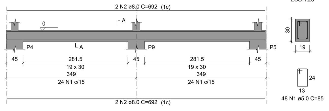
Vb4 ESC 1:50
