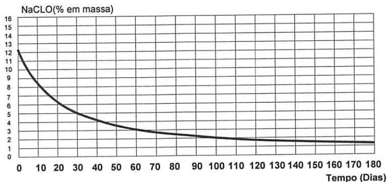
Gráfico 2: Decomposição em Função da Temperatura (Concentração Inicial: 12% NaClO - Temperatura 40°C)
