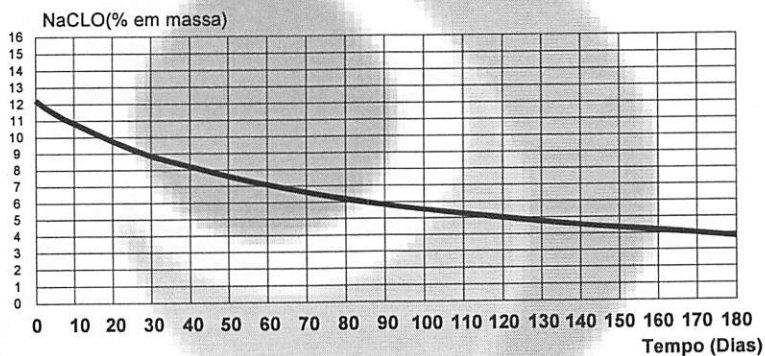
Gráfico 1: Decomposição em Função da Temperatura (Concentração Inicial: 12% NaClO - Temperatura 30°C)
